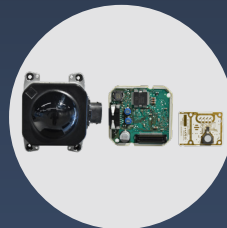
Radars
